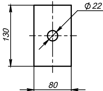
Поз.2 (Накладка)
